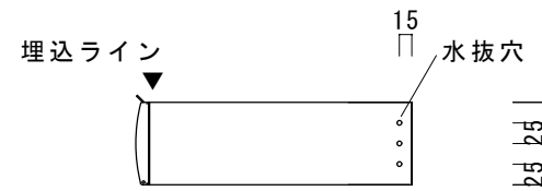
底面
