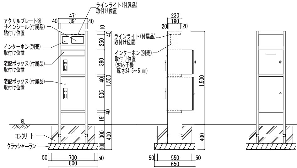
(側面図)
