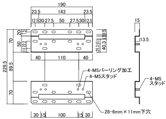
●ポスト取付けベース ビス穴位置
