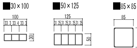
(断面図)
