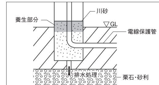
排水処理<コンクリート基礎の場合>
