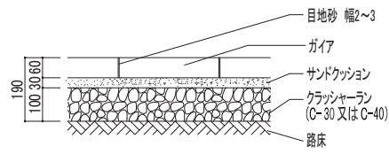
歩掛表 (100 m 2 当り)
