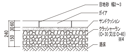
歩掛表 (100 m 2 当り)
