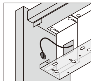
②-4 インターホンの厚みに合わせてビス固定します
