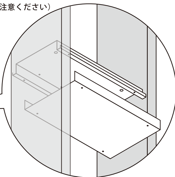
ポスト台座の 下面パネルを外します
