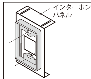
②-1 インターホンパネルにフレームを固定します
