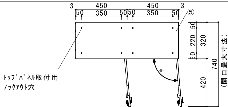
943.6 (開口最大寸法) 天面
