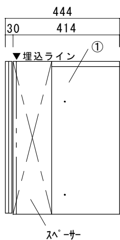
右側面
