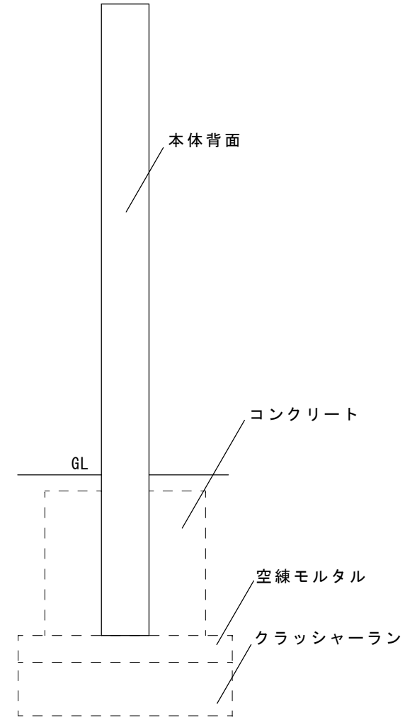
背面
