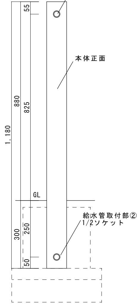
正面
