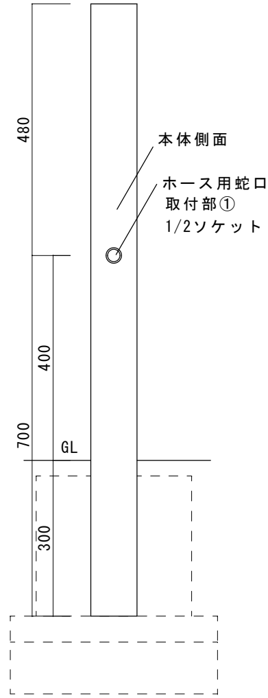
右側面
