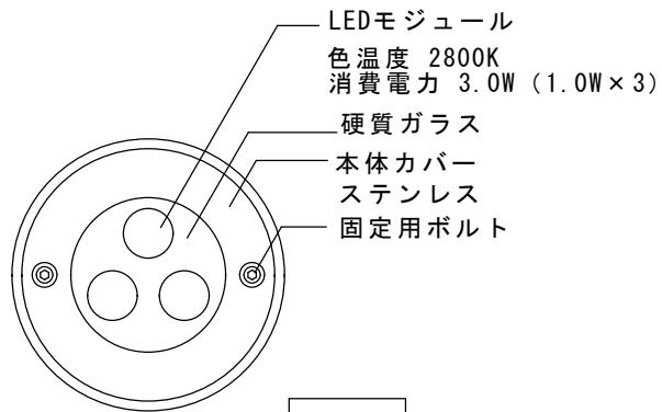
天面
