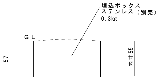
埋込断面
