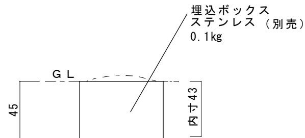
埋込断面
