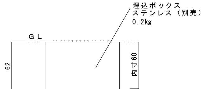
埋込断面
