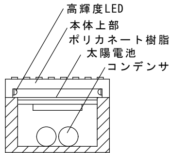
断面
