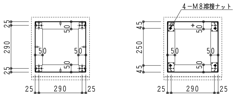
アンカー図
