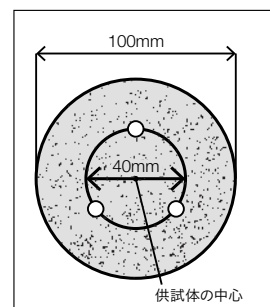
図10.14 熱電対の設置位置図
