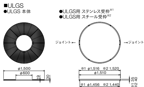
■参考施工図(mm)
