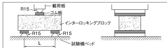
図10.1 試験装置
