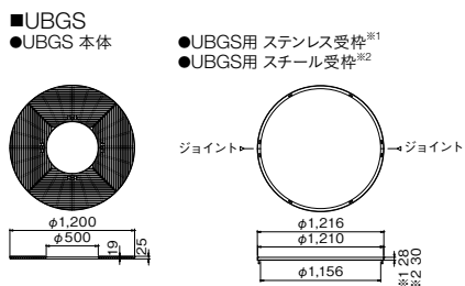
■参考施工図(mm)
