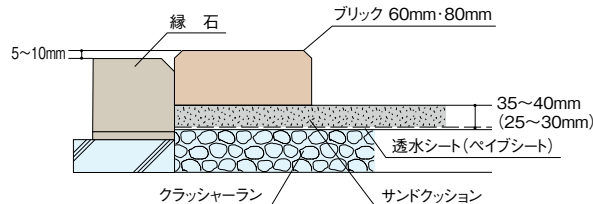
(図-1) サンドクッション転圧前
