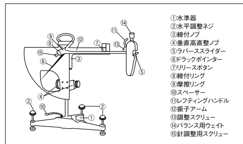
図10.8 ポータブルスキッドレジスタンステスター
