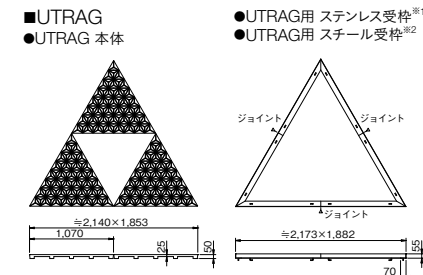
■参考施工図(mm)
