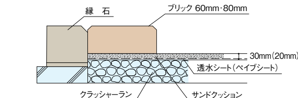
(図-2) サンドクッション転圧後
