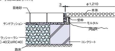
■参考施工図(mm)
