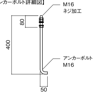
【アンカーボルト詳細図】
