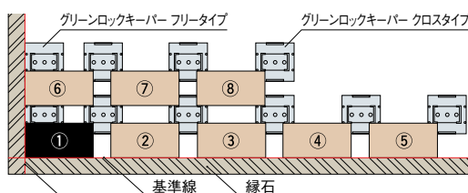
(図-3) グリーンロックキーパーとブリックの敷設順序
