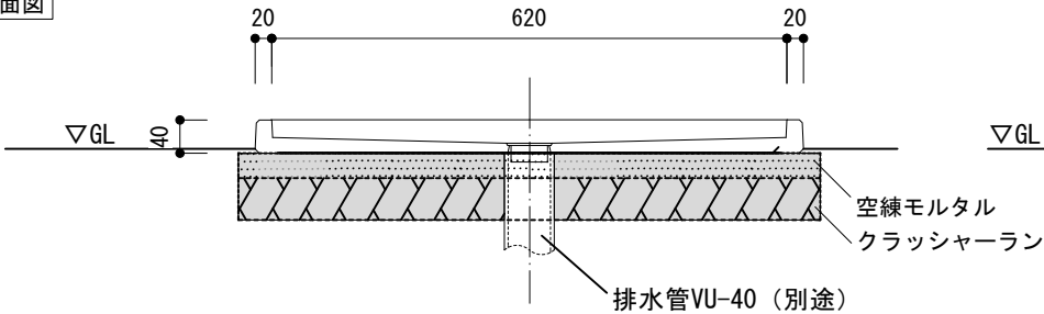
断面図
