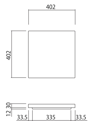
シートトップ
