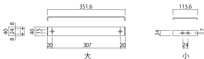
シートトップ取付金具
