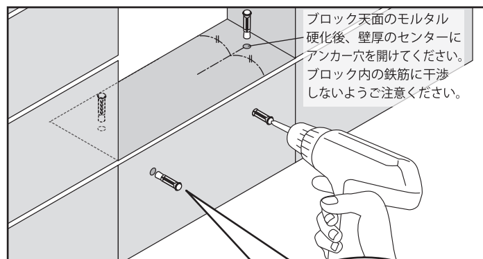
② コンクリートに下穴を開け、オールプラグボルトを取り付けます。(4ヶ所) 下穴：φ11mm 深さ40mm
