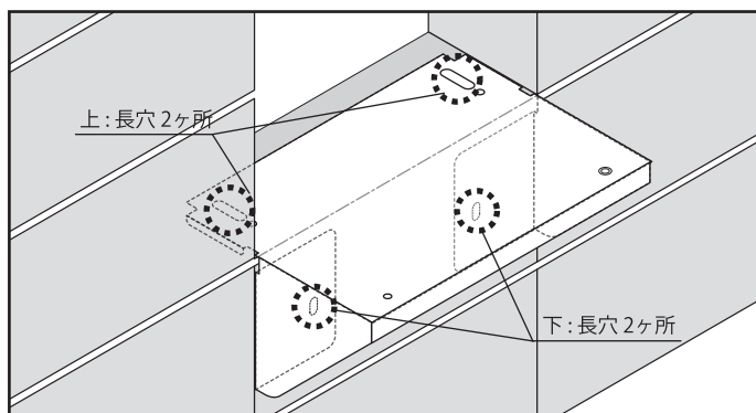
① 台座を仮置きし、穴位置をマーキングします。(4ヶ所)
