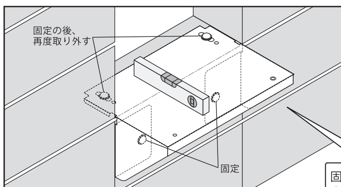
③ 水準器で確認しながら固定します。 (ビスは本体取付後に増し締めします。) 水平が出ていない場合は下地を調整してください。
