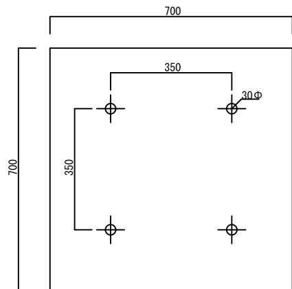
底面図
