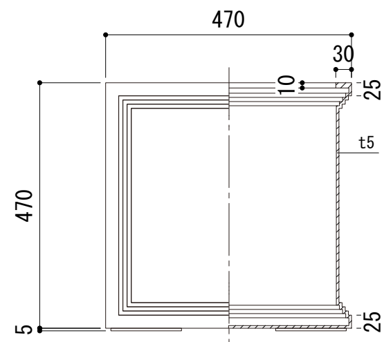
側・断面図
