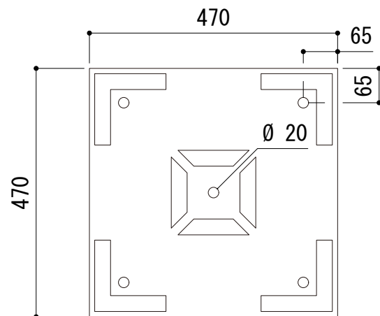
底面図
