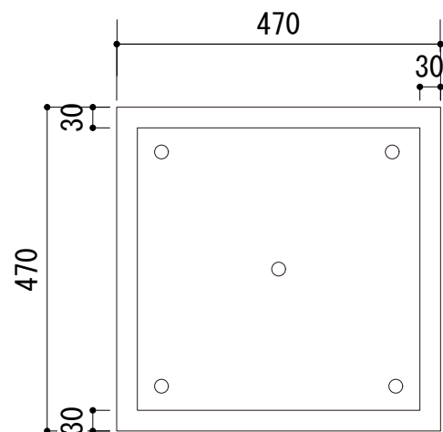
平面図
