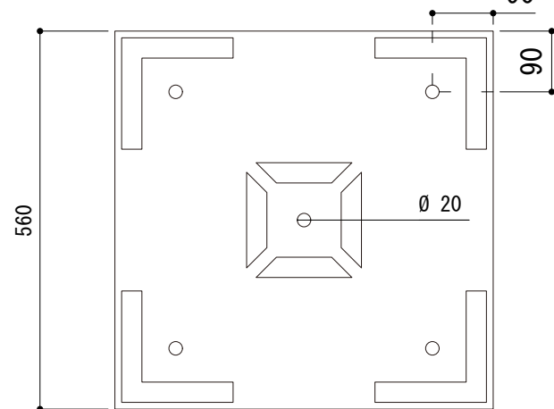
底面図
