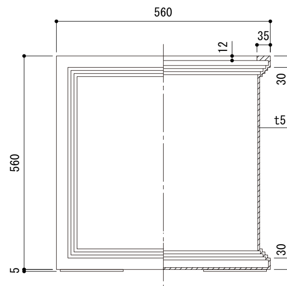
側・断面図
