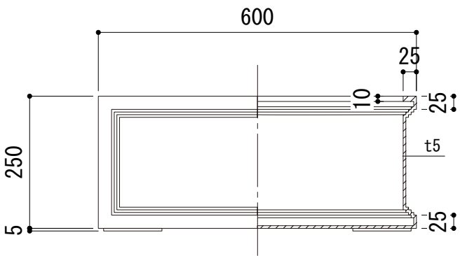
立・断面図
