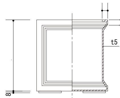
側・断面図
