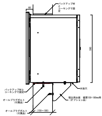
■ディコススマート08 埋込みタイプ (壁厚150-180mm) 100ポスト有り / 120ポスト無し 共通
