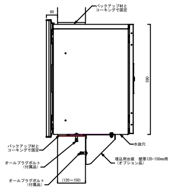
■ディコススマート08 埋込みタイプ (壁厚120-150mm) 100ポスト有り / 120ポスト無し 共通
