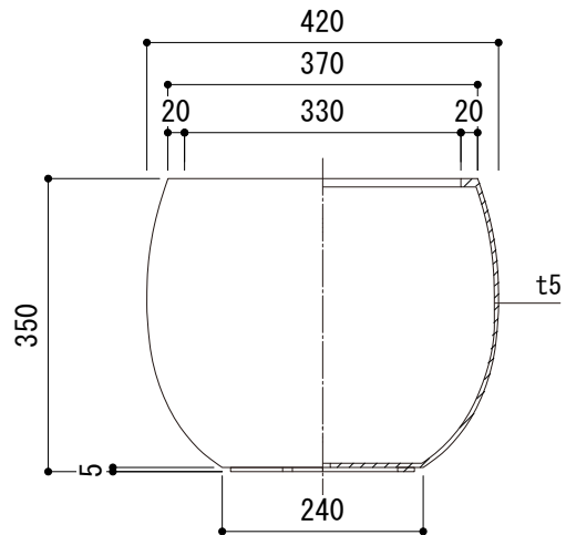
立・断面図
