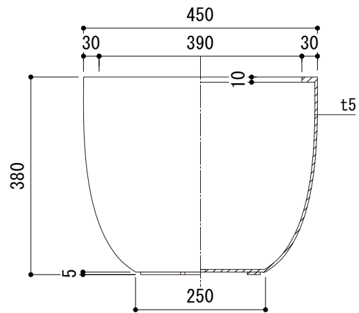
立・断面図
